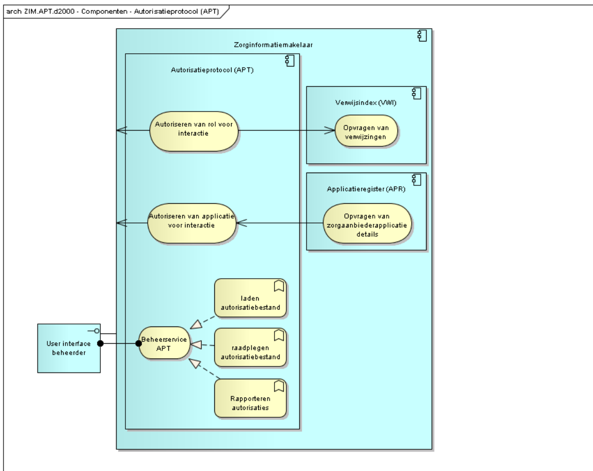
Diagram ZIM.APT.d2000 Context van het autorisatieprotocol
