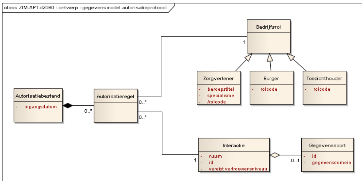
Diagram ZIM.APT.d2050 Gegevensmodel (Technisch) Autorisatiebestand
