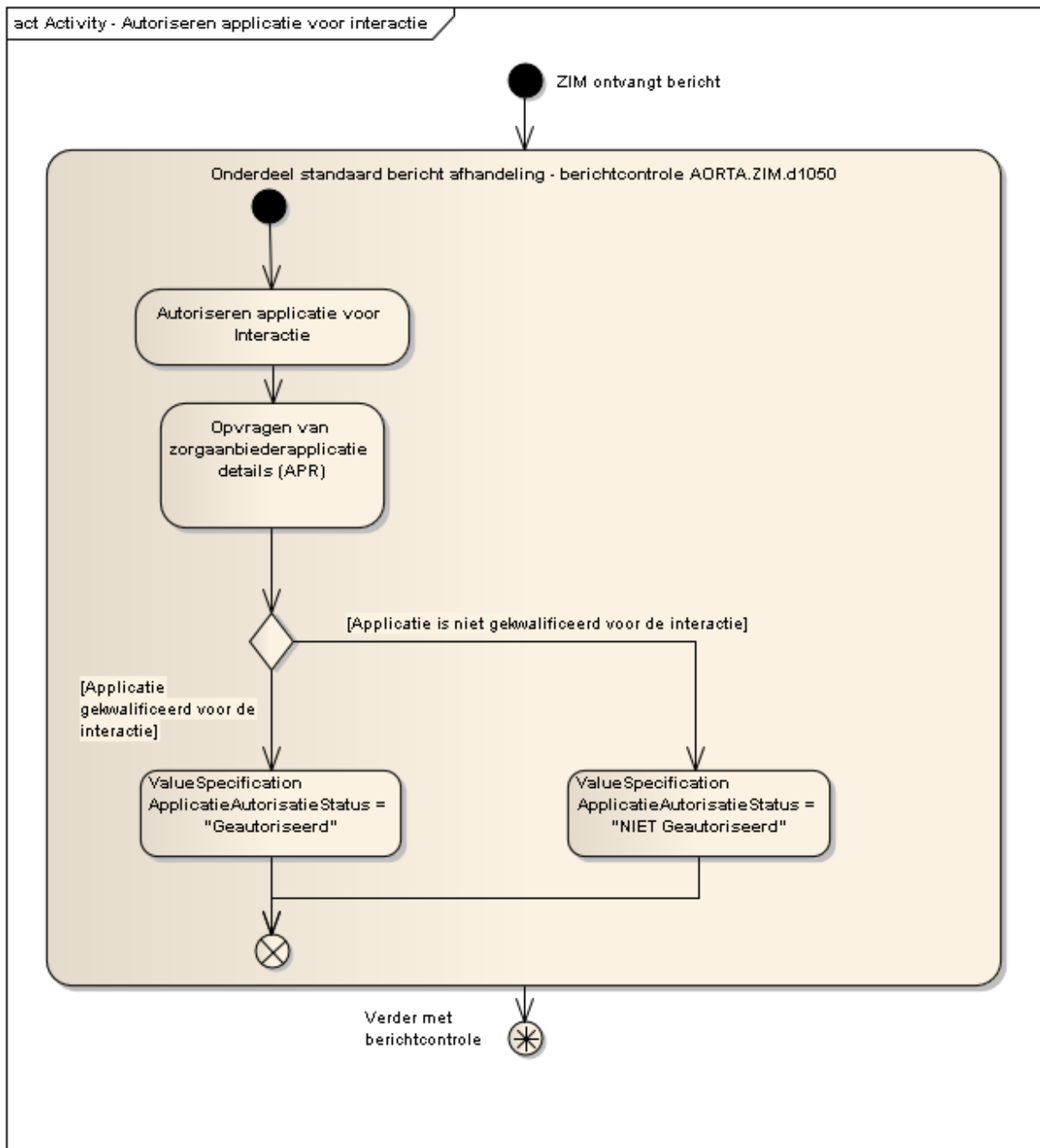
Diagram ZIM.APT.d2040 Activity Autoriseren applicatie voor interactie.
